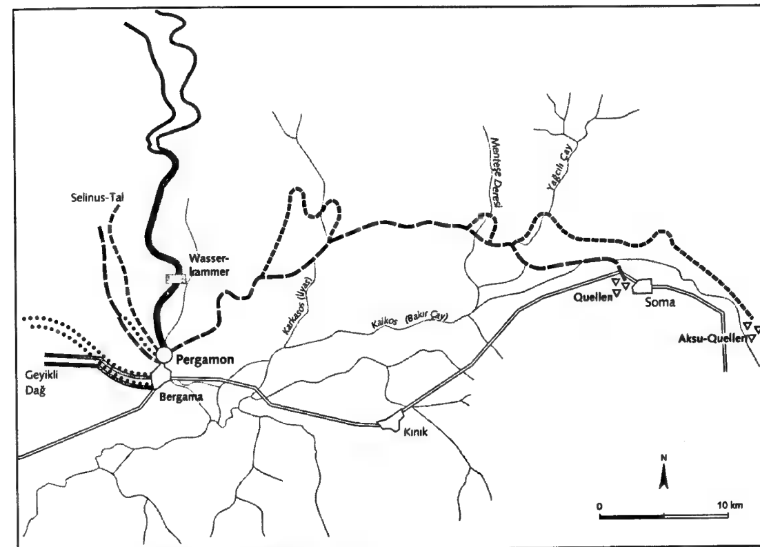
Abb. 2: Pergamon, Verlauf der Wasserleitungen (Übersichtsplan).
